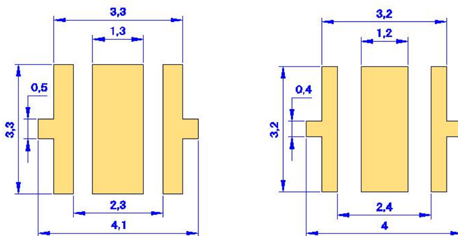
建议焊盘图
