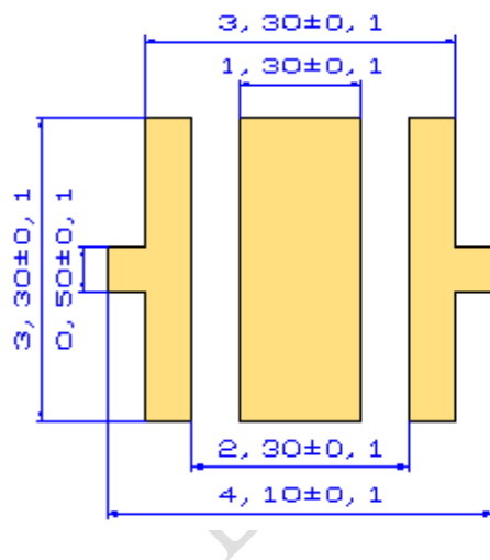
建议 PCB 焊盘
