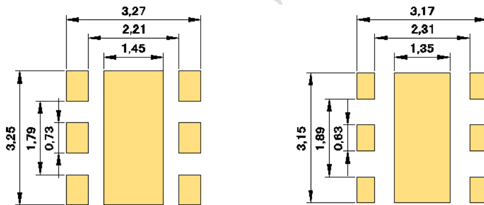
建议焊盘图
