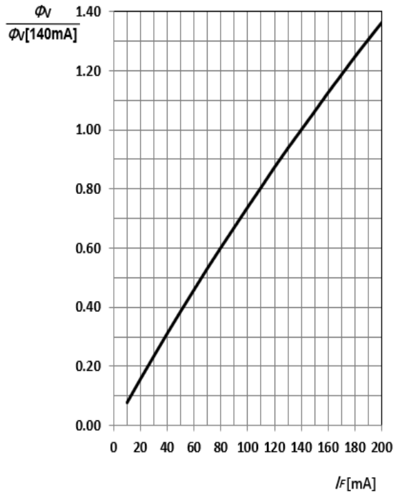
Fig 4. 相对发光强度 Relative Luminous Flux
